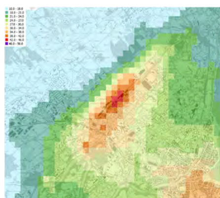
Figure 12 : Immissions moyennes annuelles de NO 2 , état de référence 2017 [µg/m 3 ].
