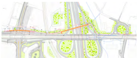
Avant-projet passerelle le long de la route de Meyrin (Kung ingénieurs – OCGC, 2018).
