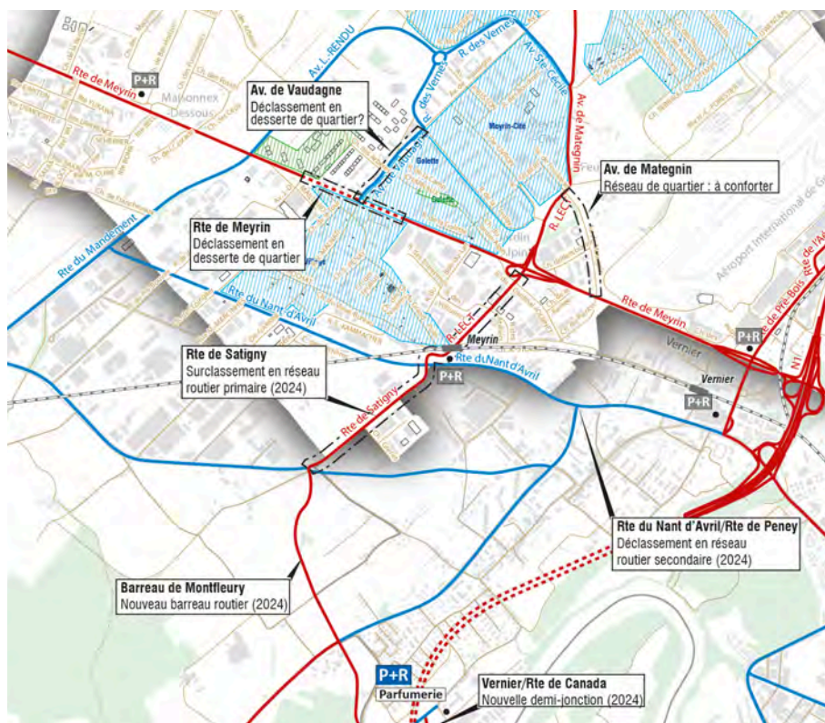
Fig. 14 : Hiérarchie du réseau routier (état 2025) : barreau de Montfleury – rue Lect – avenue de Mategnin (rgr)
