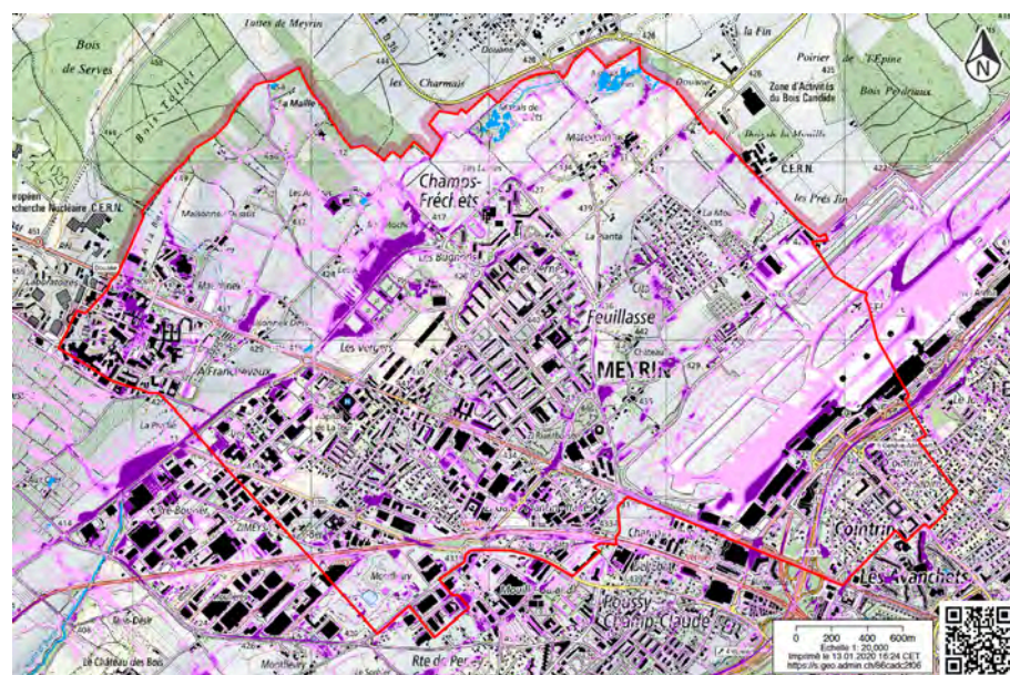
Fig. 9 : Carte de l'aléa de ruissellement (OFEV)
