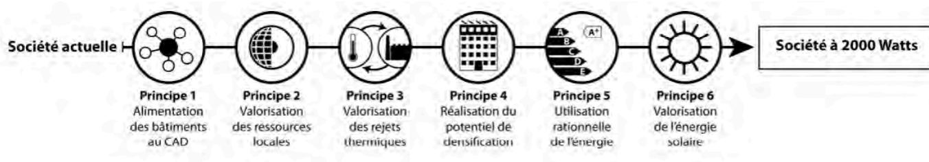
Fig. 34 : Six principes pour tendre vers la Société à 2000 Watts (CGSE, 2019)
