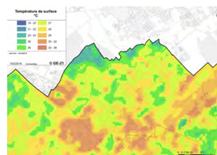
Température des surfaces sur la commune de Meyrin (Schlaepfer, Guinaudeau et al., 2018 (Projet NOS-ARBRES)).
