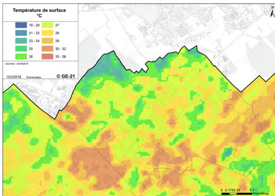
Fig. 11 : Température des surfaces sur la commune de Meyrin. Source : Schlaepfer, Guinaudeau et al. (2018). Projet NOS-ARBRES
