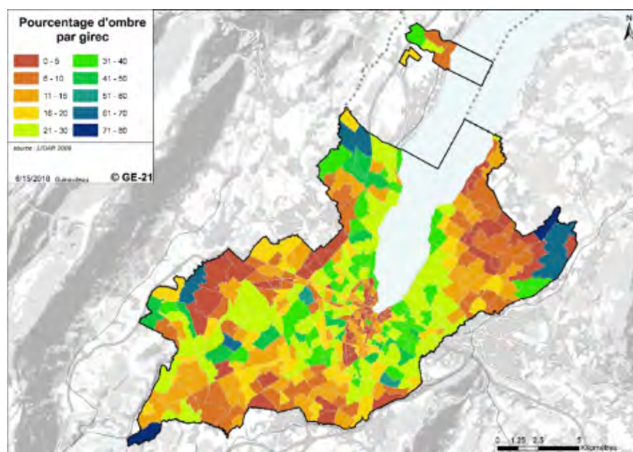
Fig. 10 : Pourcentage d'ombre au sol au niveau cantonal. Source : Schlaepfer, Guinaudeau et al. (2018). Projet NOS-ARBRES
