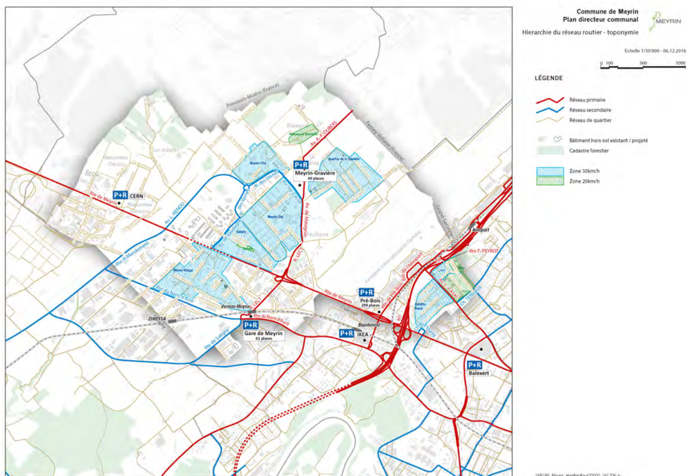
Fig. 16 : Hiérarchie du réseau routier, état actuel 2019
