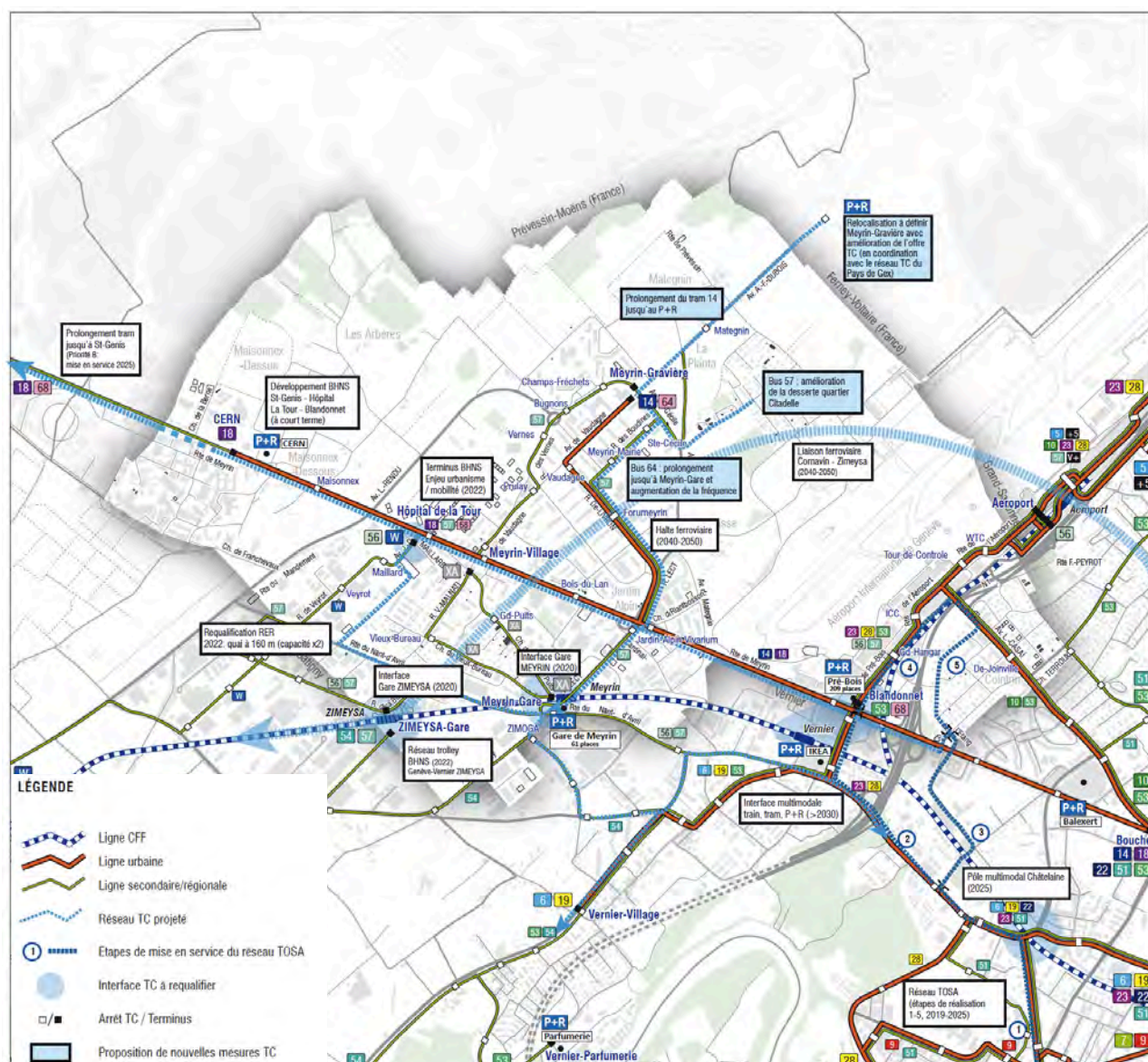
Fig. 21 : Hiérarchie du réseau TC, état futur
