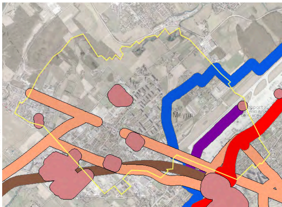
Fig. 8 : Impact territorial de l'OPAM (SITG)
