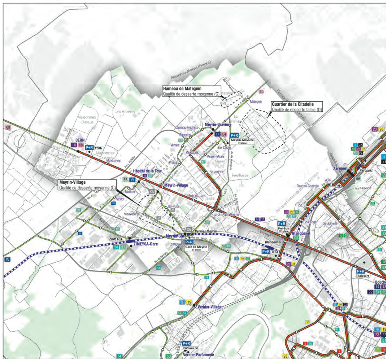
Fig. 19 : Réseau actuel des transports publics
