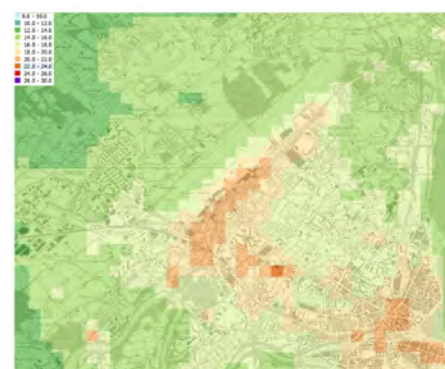
Figure 15 : Immissions moyennes annuelles de PM 10 , prévisions 2022 [µg/m 3 ].
