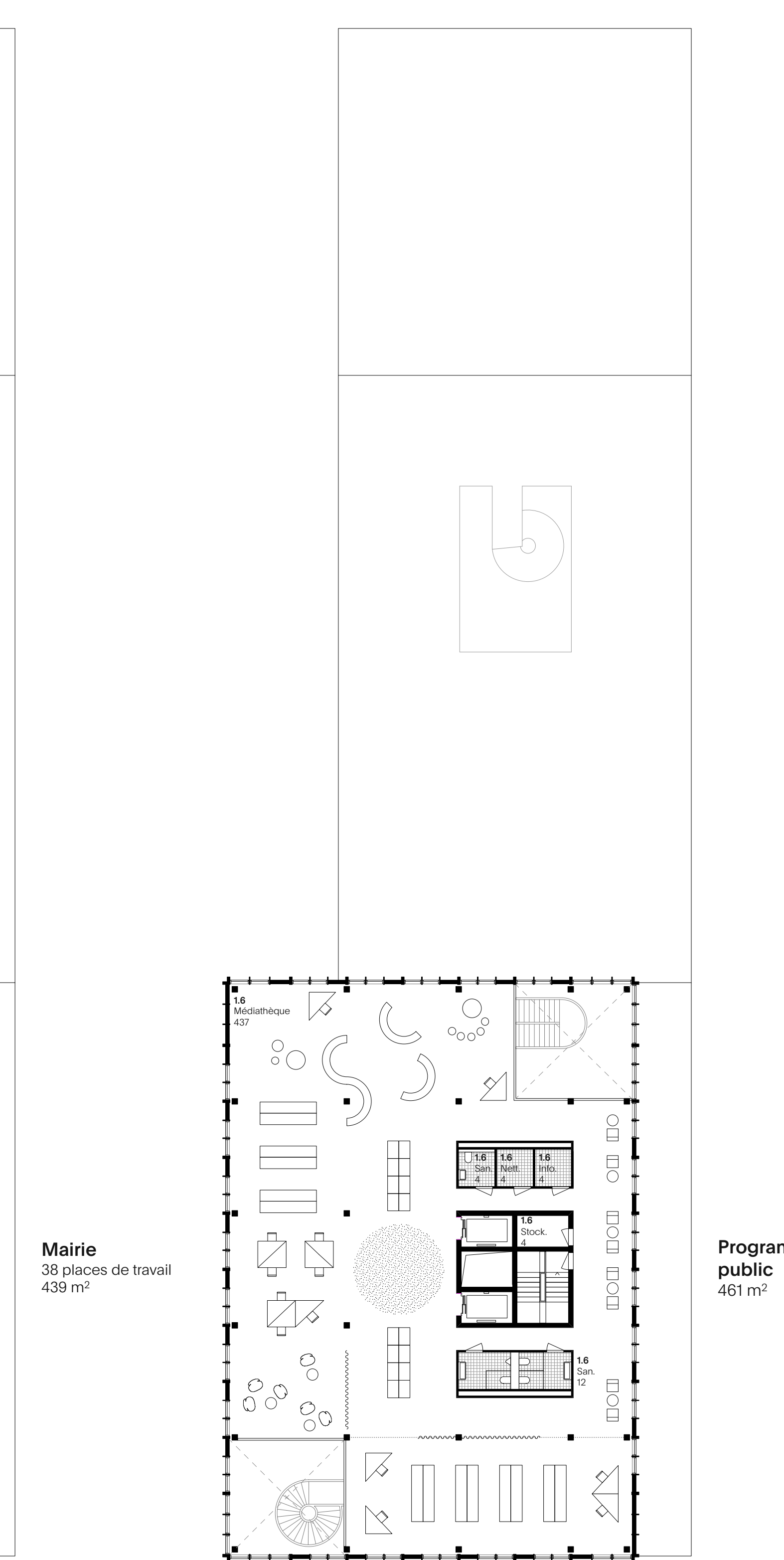
Plan du 6 e étage 1 / 200
