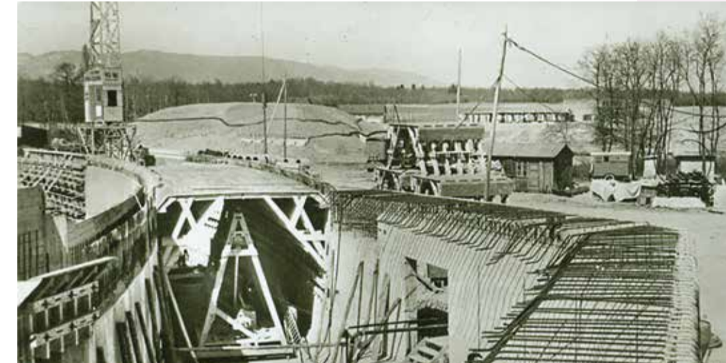
Construction du CERN, fin des années 50. L'anneau. Carte postale, collection Ch. Noir.
